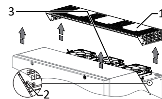
Abb. 76: Abdeckung entfernen
