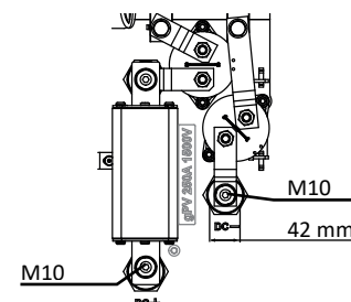
Abb. 23: DC-Anschluss XL-Version
