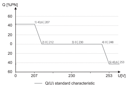
Abb. 55: Q(U) Standard Kennlinie mit 5 Stützstellen
