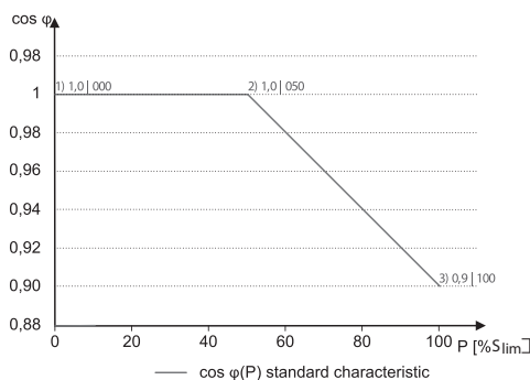
Abb. 54: \cos \varphi(P) Standard Kennlinie mit 3 Stützstellen
