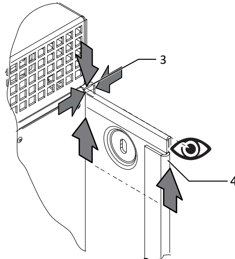
Abb. 14: Gerät in Halterung einhängen
