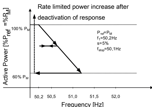
Abb. 63: Beispielverhalten mit Hysteresis (Modus 1)
