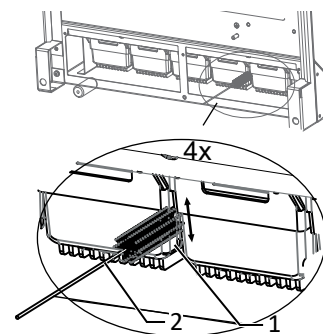
Abb. 75: Kühlrippen von unten reinigen
