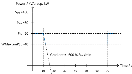
Abb. 71: Leistungsgradient gemäß Musterparameter und Berechnung
