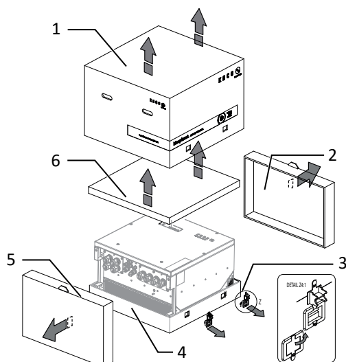
Abb. 9: Kartontage öffnen
