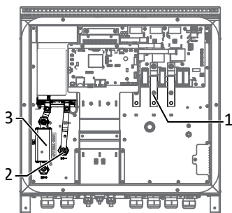
Abb. 16: Anschlussbereich M-Version
