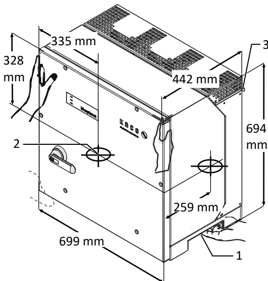
Abb. 13: Gerät am Eingriff anheben
