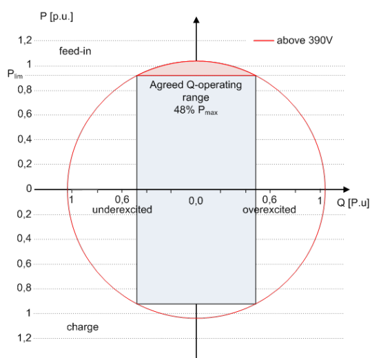
Abb. 70: P-Q-Betriebsbereich mit begrenzter Wirkleistung ( Q_{max}=S_{max}\neq P_{max} ) Speicherwechselrichter
