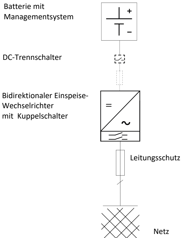
Abb. 4: Übersichtsschaltplan für eine Anlage mit einem Bidirektionaler Einspeise-Wechselrichter
