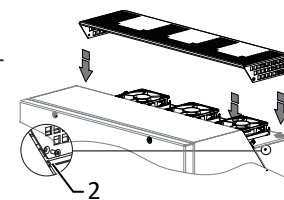
Abb. 80: Abdeckung aufsetzen
