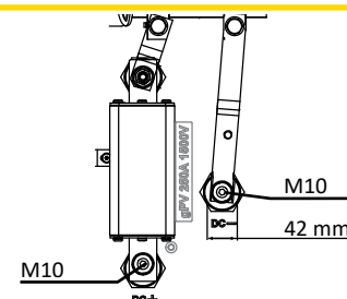
Abb. 24: DC- Anschluss M-Version
