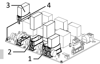
Abb. 25: AC-Überspannungsschutz nachrüsten
