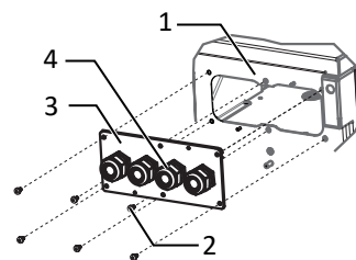
Abb. 19: AC Eingangsplatte lösen
