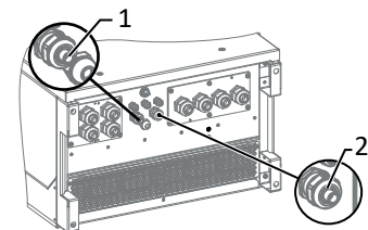
Abb. 29: Signalleitungen einföhren
