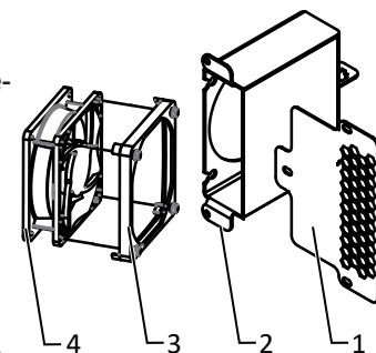
Abb. 79: Innenraumlüfter lösen
