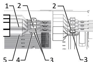
Abb. 20: AC-Anschluss vorbereiten
