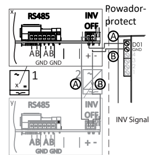
Abb. 30: Gerät mit Powador-Pro- tect verbinden
