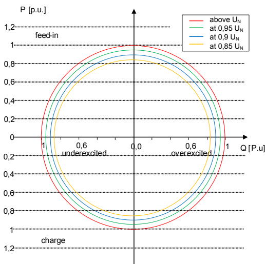
Abb. 48: P-Q Betriebsbereich für bp gridsave 92.0 TL3-S
