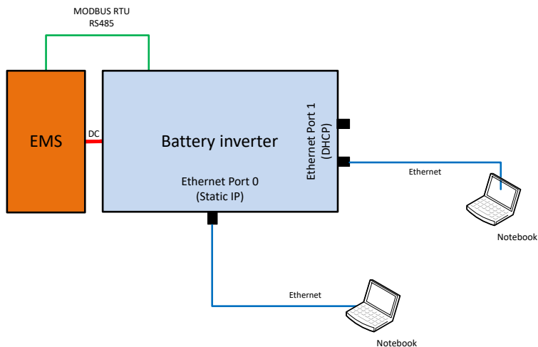
Abb. 35: Inbetriebnahme über Ethernet
