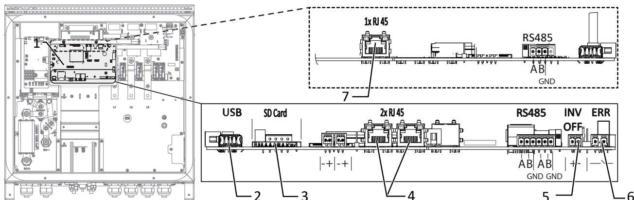
Abb. 28: Kommunikationsplatine (HMI-Platine)
