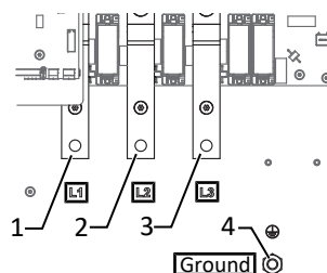
Abb. 21: AC-Netzanschluss 4-polig
