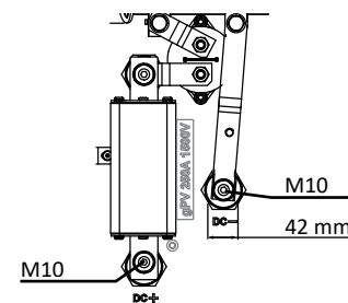
Abb. 22: DC-Anschluss L-Version
