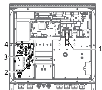
Abb. 18: Anschlussbereich XL-Version
