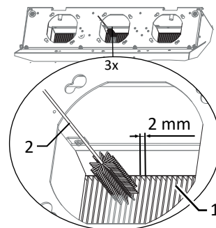
Abb. 74: Kühlrippen von oben reinigen
