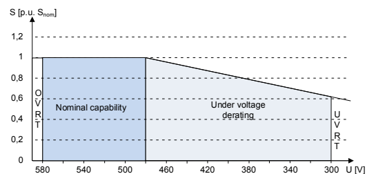
Abb. 49: Scheinleistung abhängig der Netzspannung für gridsave 92.0 TL3-S
