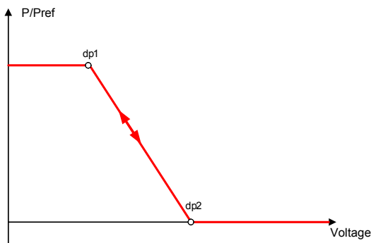
Abb. 57: Beispiel-Kennlinie ohne Hysterese
