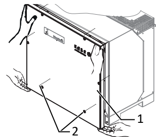
Abb. 15: Gehäusedeckel abnehmen
