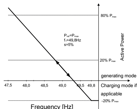
Abb. 64: Beispielverhalten ohne Hysteresis (Modus 2) Zum Zeitpunkt der Aktivierung befindet sich der Wechselrichter im Ladebetrieb mit 20 % Ladeleistung.
