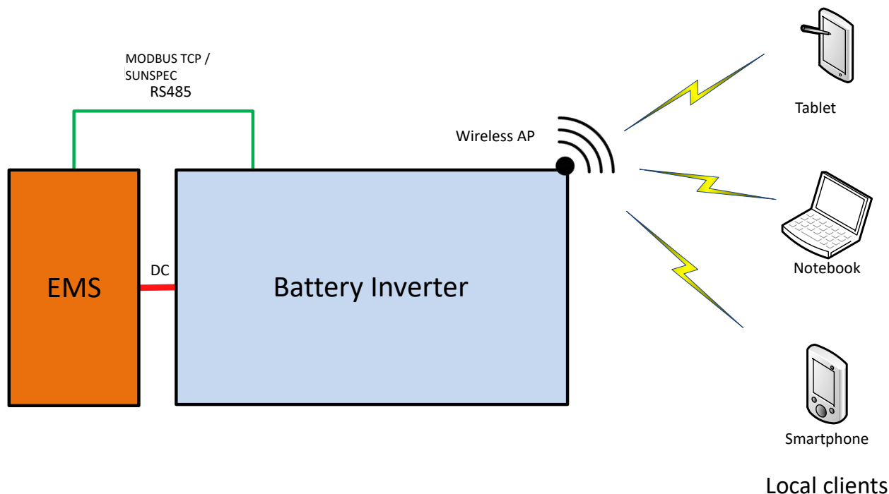
Abb. 33: Inbetriebnahme über WIFI Direktverbindung
