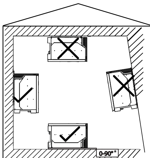
Abb. 8: Erlaubte Aufstelllage
