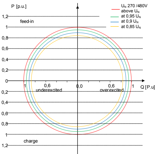
Abb. 50: P-Q Betriebsbereich für bp gridsave 110 TL3-S
