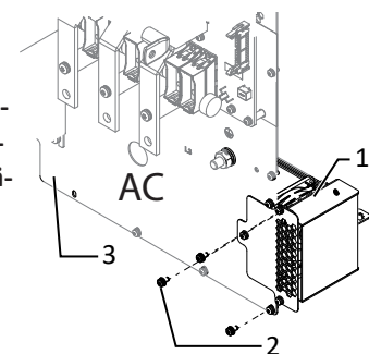
Abb. 78: Innenraumlüfter ausbauen
