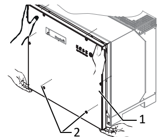
Abb. 32: Gehäusedeckel schließen
