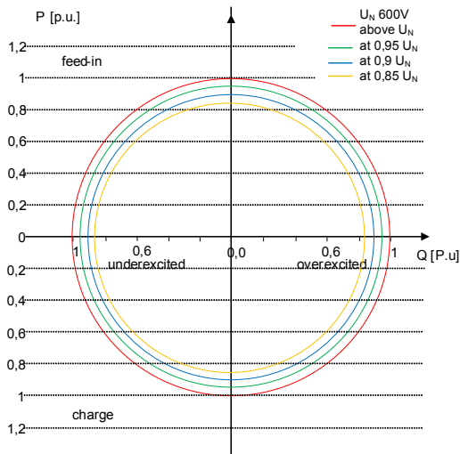
Abb. 52: P-Q Betriebsbereich für bp gridsave 137 TL3-S
