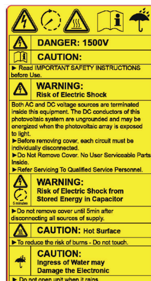
Abb. 2: Warnetikett
