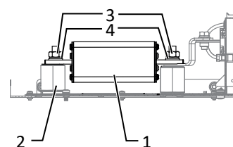
Abb. 81: DC-Sicherung ersetzen
