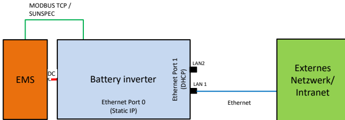
Abb. 36: Inbetriebnahme über externes Netzwerk
