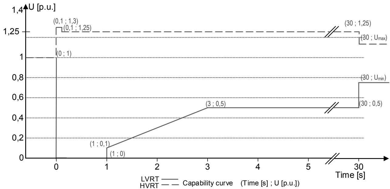
Abb. 65: Störfestigkeitskennlinie bezogen auf die Nennspannung
