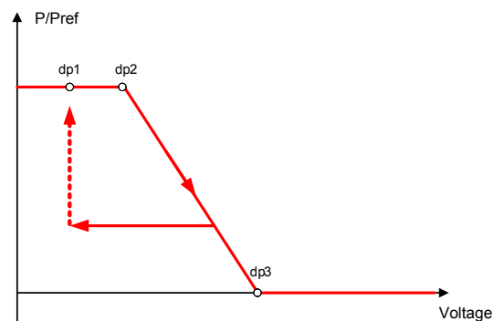
Abb. 58: Beispiel-Kennlinie mit Hysterese und einer Deaktivierungsschwelle unterhalb der Aktivierungsschwelle
