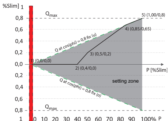
Abb. 56: Q(P) Standard Kennlinie mit 5 Stützstellen
