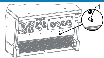
Abb. 27: Zusätzlicher Erdungspunkt 1 Erdungsbolzen
