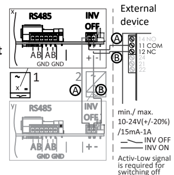
Abb. 31: Gerät mit externem Netzschutzgerät verbinden
