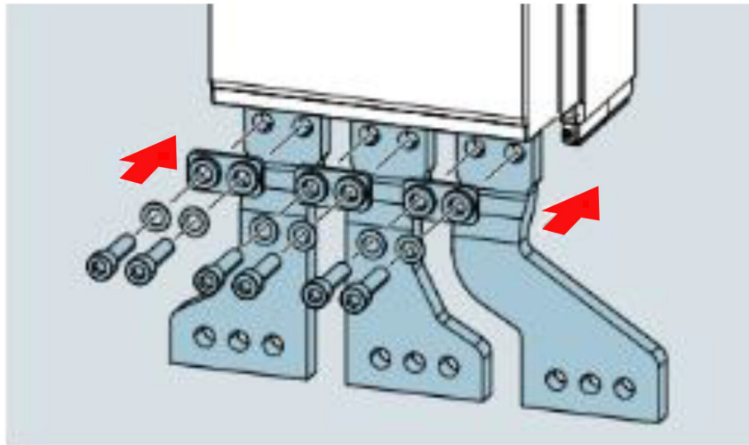
Abbildung 1. Hauptanschlüsse — Kompaktleistungsschalter
