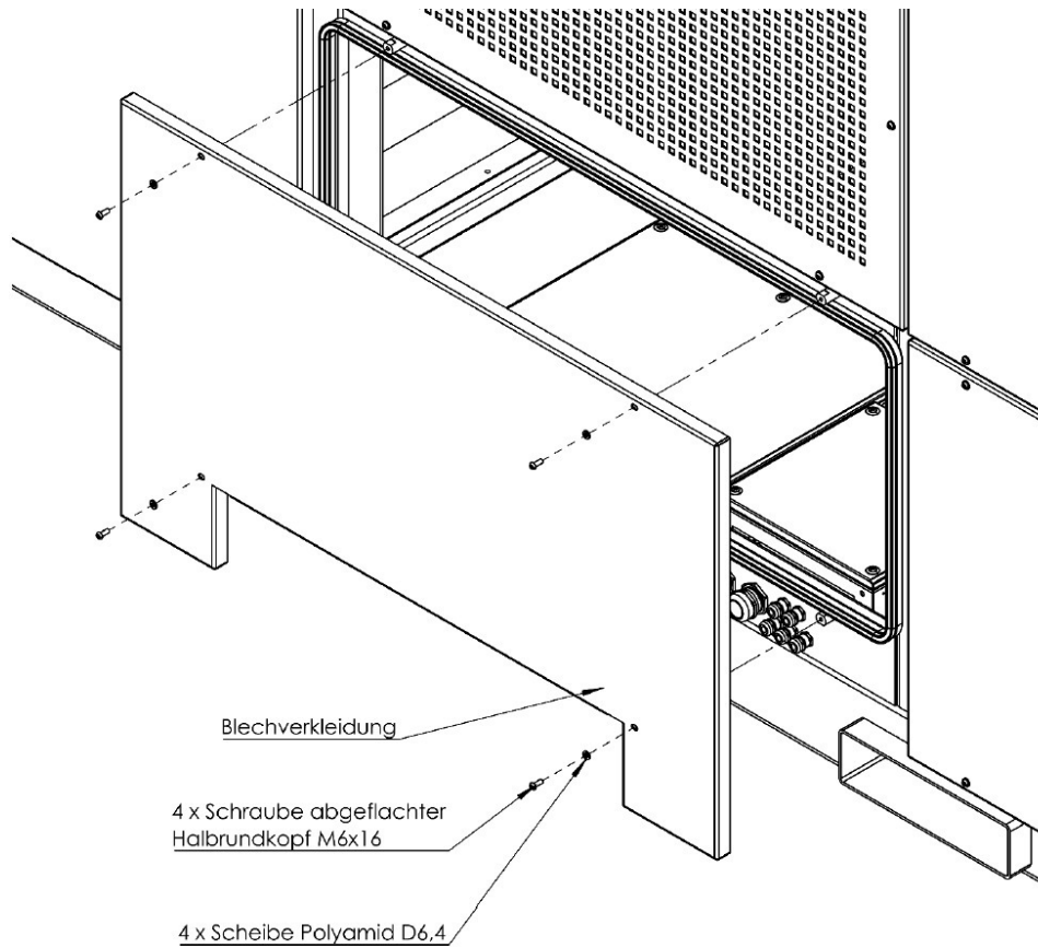
Abbildung 25. Demontage — Abdeckblech für Verkabelung
