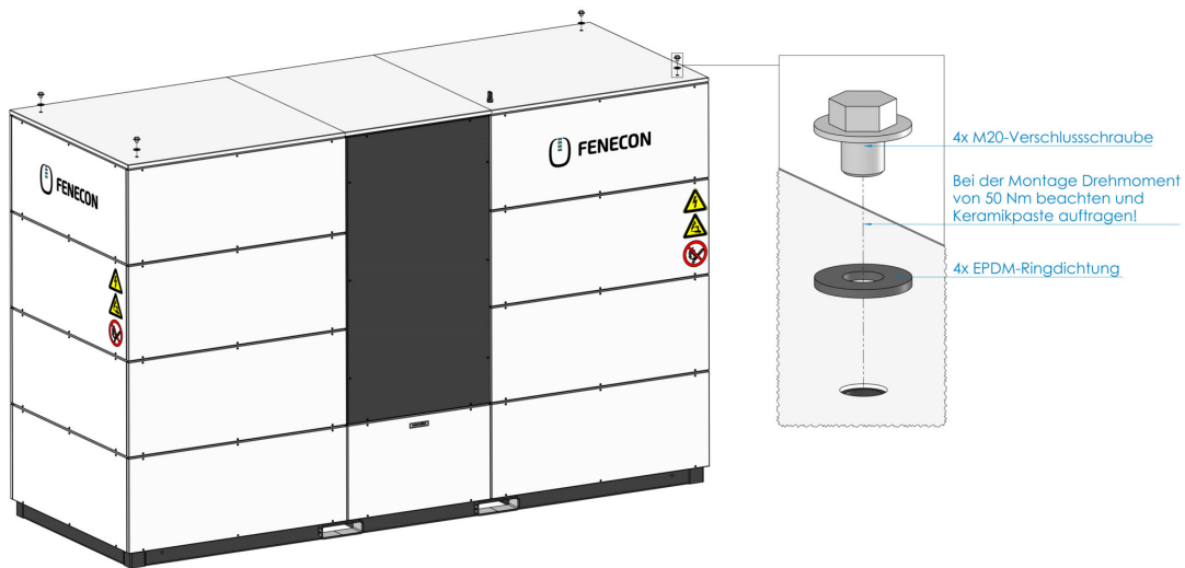
Abbildung 22. Montage der Dichtungen
