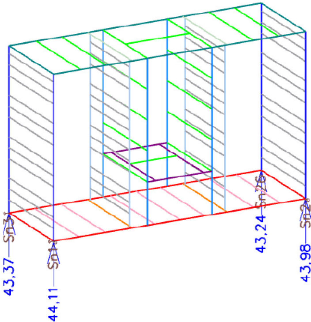
Abbildung 16. Auflagerreaktionen — Container
