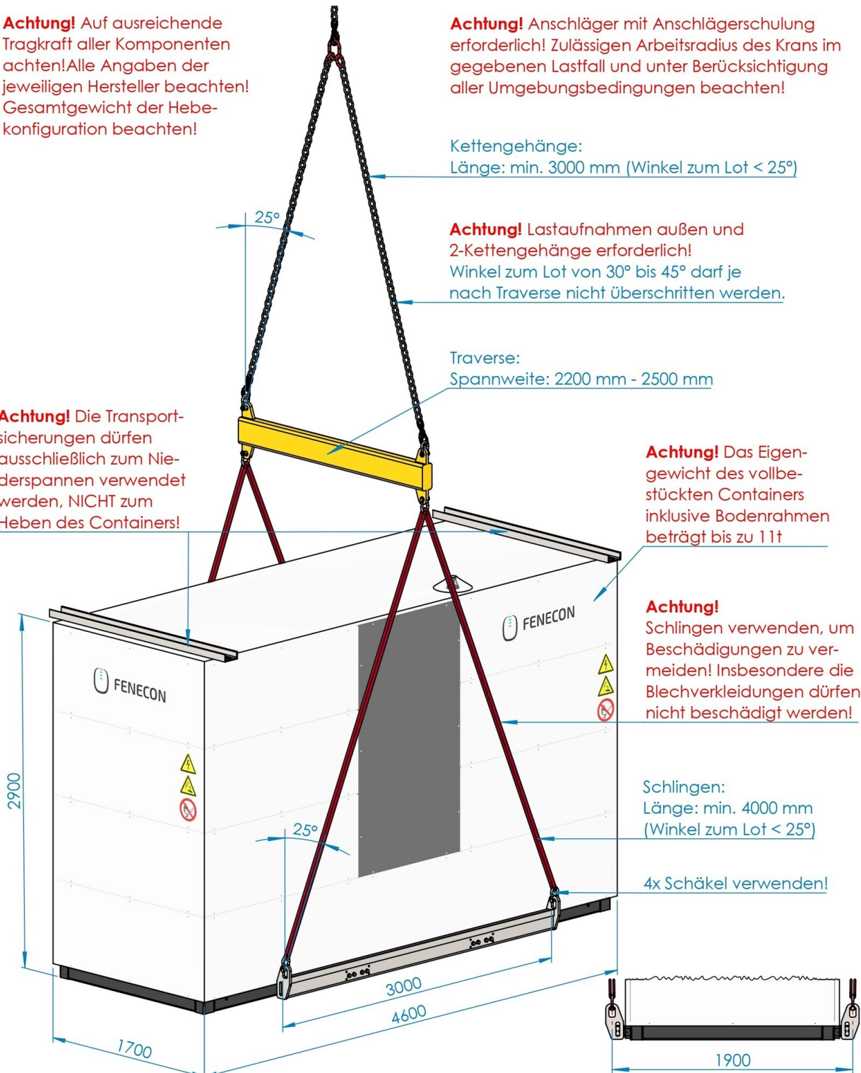
Abbildung 19. Hebeanweisung für fertig bestückte Variante
