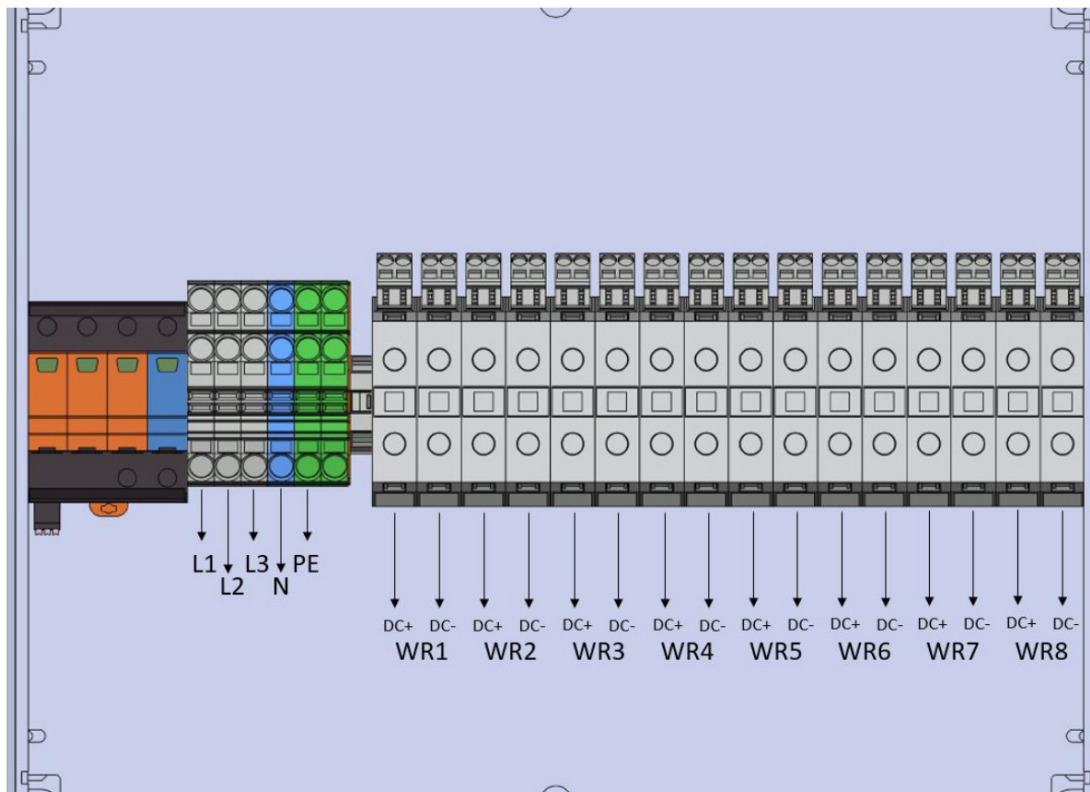
Abbildung 13. Komponenten in DC-/AC-Anschlussbox
