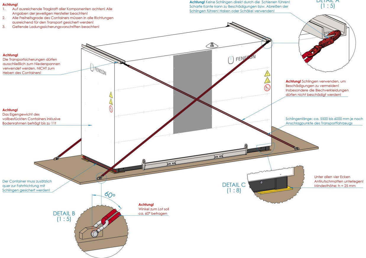
Abbildung 18. Transportsicherung für fertig bestückte Variante
