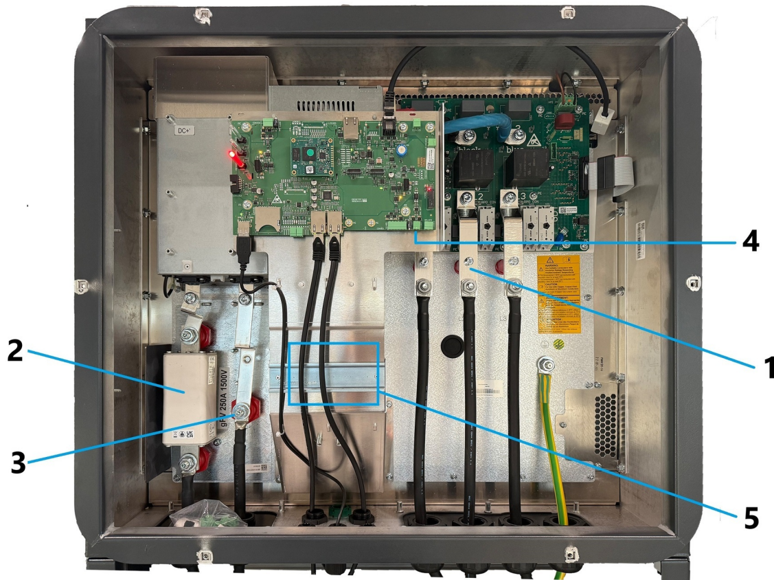
Abbildung 12. Anschlussbereich – Wechselrichter
