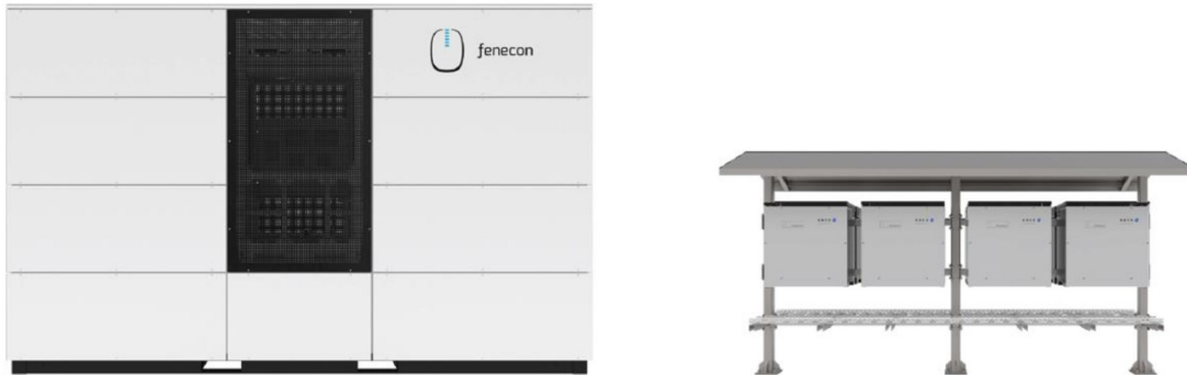
Abbildung 3. FENECON Industrial L mit Wechselrichtergestell
