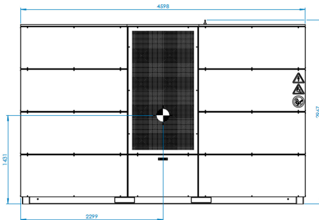
Abbildung 7. Abbildung von vorne mit Bemaßung und Lage des Schwerpunkts [in mm]
