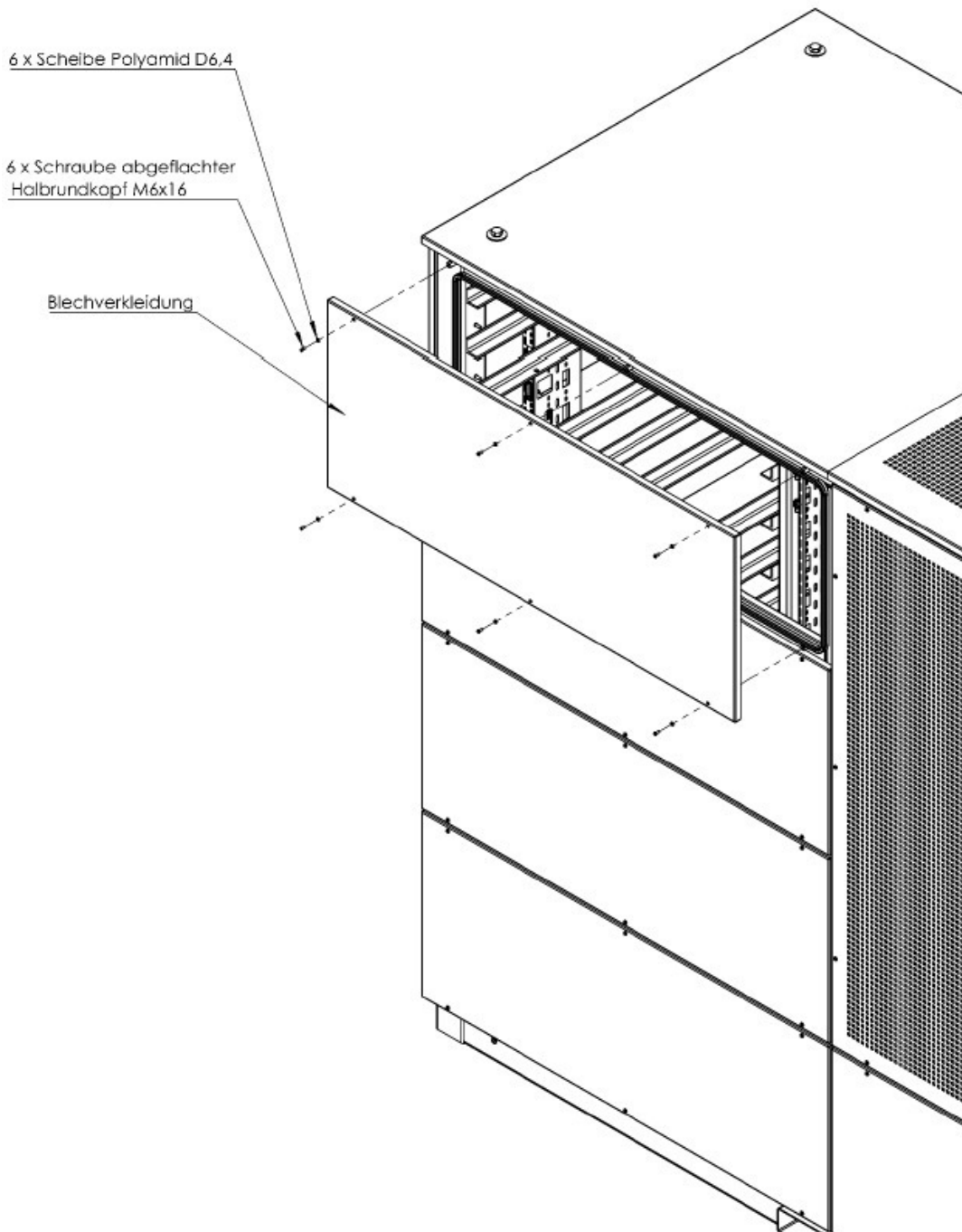
Abbildung 23. Demontage – Abdeckbleche
