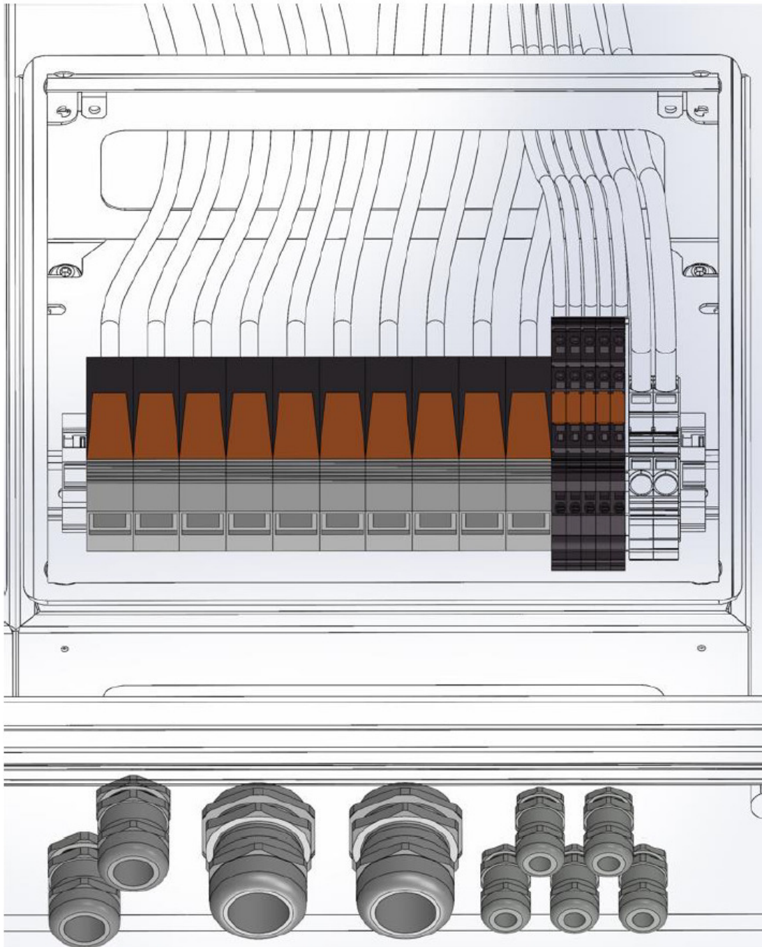
Abbildung 27. Kommunikationsverkabelung
