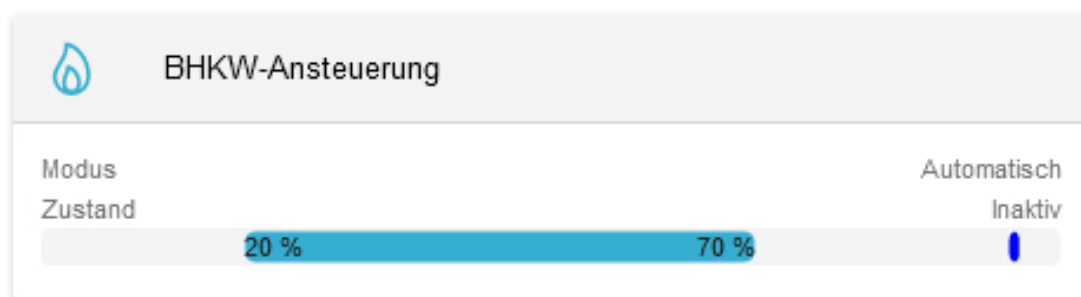
Abbildung 17. Flat-Widget
