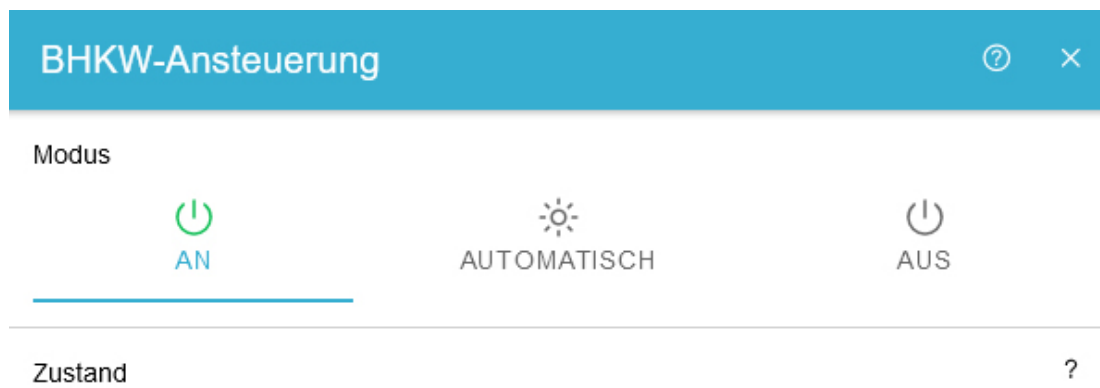
Abbildung 18. Detail-Widget
