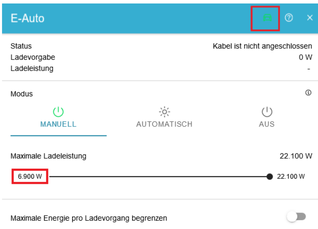
Abbildung 11. Autoverwaltung
