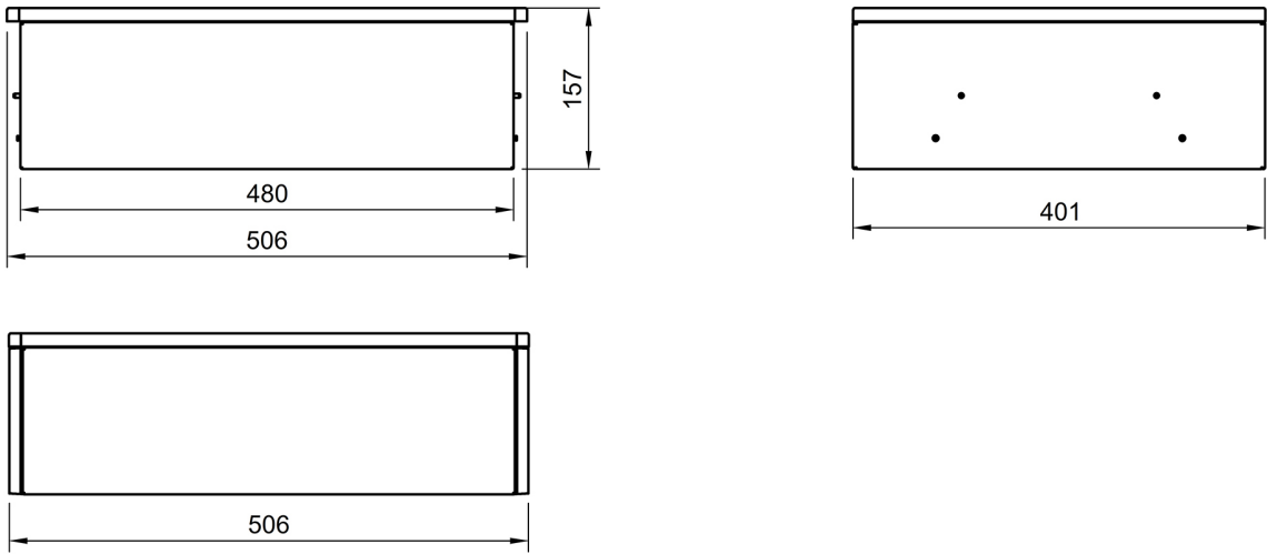
Abbildung 12. Abmessungen — Abschlussbox
