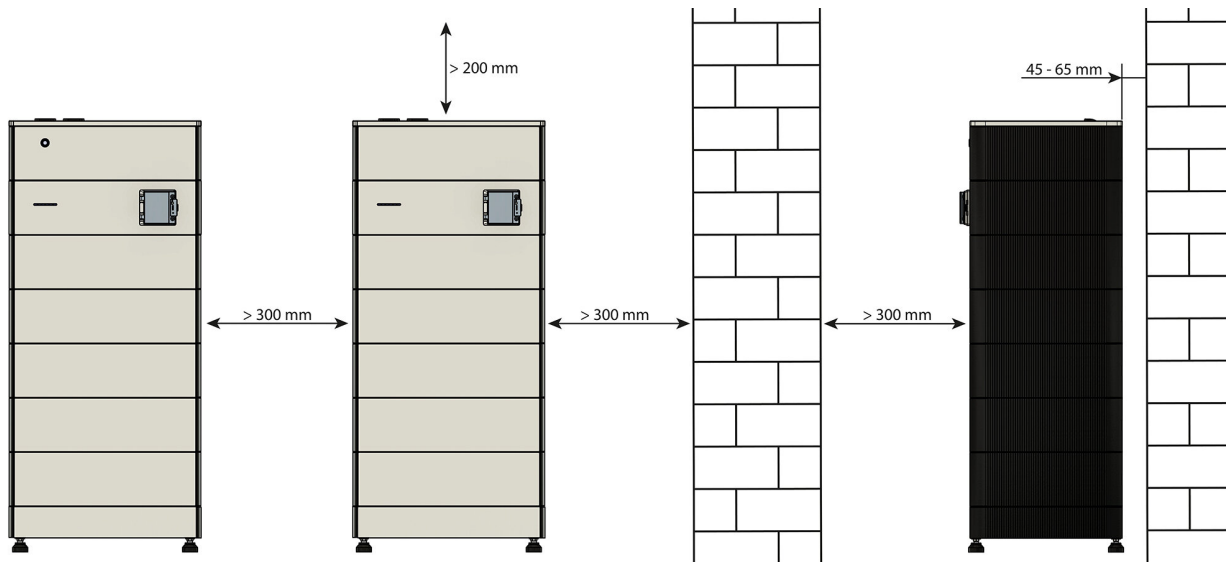
Abbildung 28. Abstände am Aufstellort
