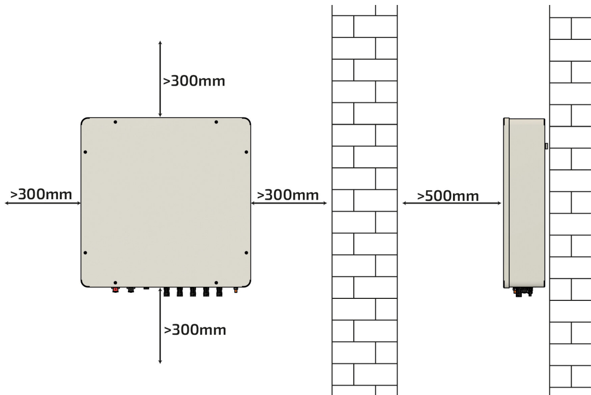
Abbildung 25. Montagebedingungen — Parallelschaltbox
