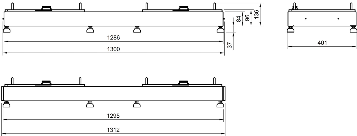
Abbildung 11. Abmessungen — Splitsockel
