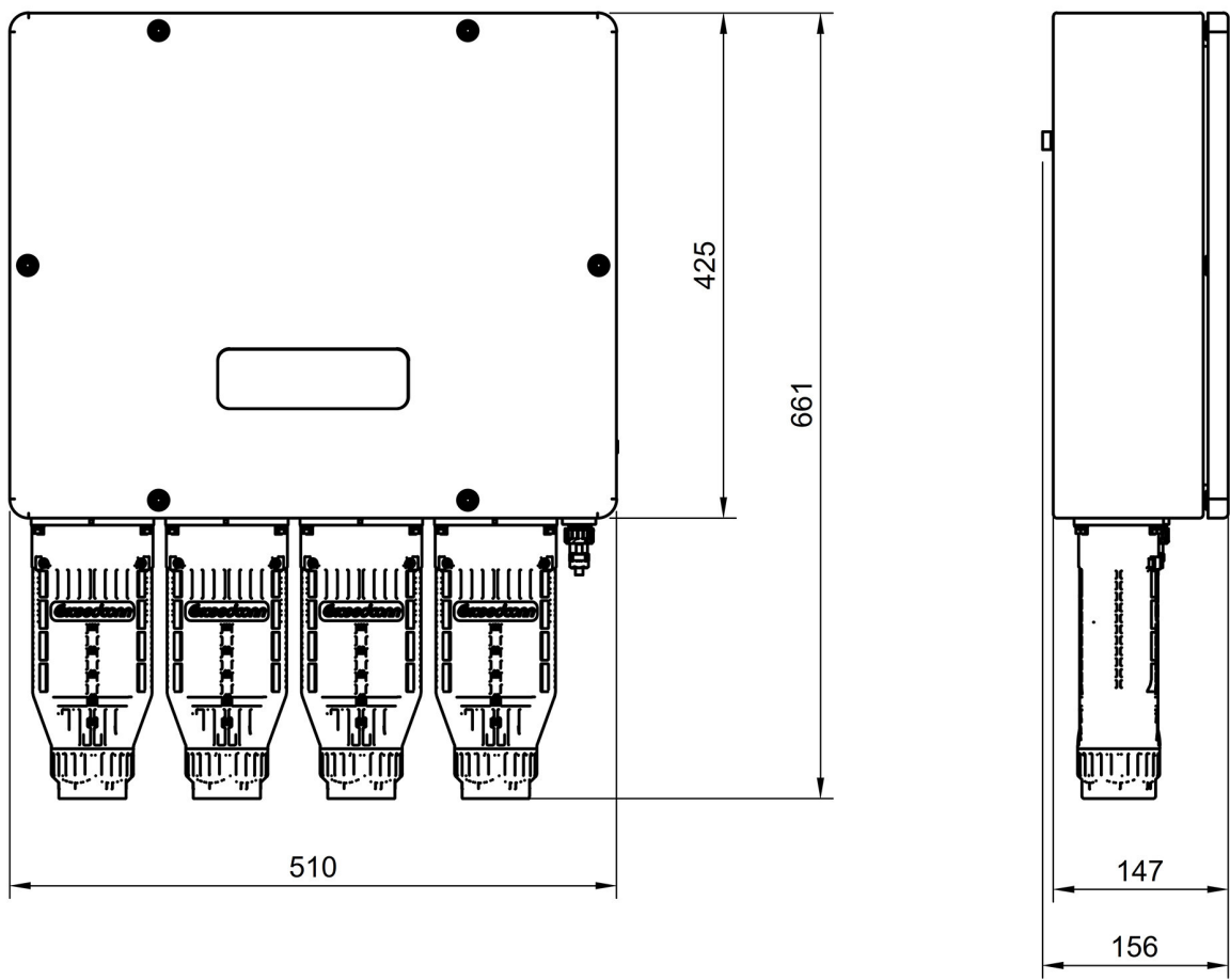
Abbildung 13. Abmessungen — STS-Box
