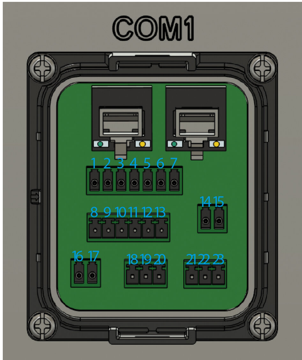
Abbildung 35. Externe Ansteuerung des Commercial-50-Wechselrichters
