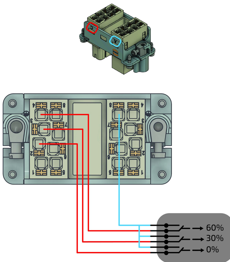
Abbildung 36. Verbindung — Rundsteuerempfänger auf NAP
