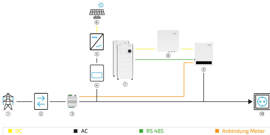
Abbildung 16. Systemaufbau als AC-System (ohne Schutzvorrichtung dargestellt)
