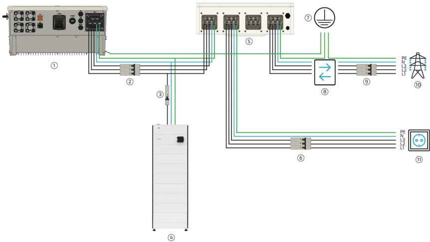
Abbildung 33. AC-Anschluss allgemein (mit STS-Box/Notstrom)
