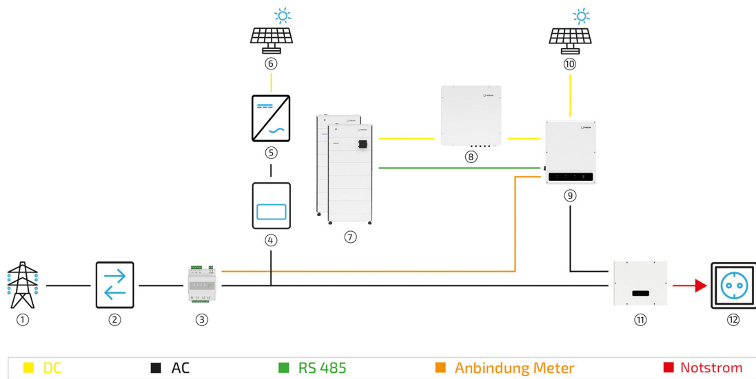
Abbildung 20. System mit STS-Notstromumschaltung und zusätzlichem PV-Erzeuger (ohne Schutzeinrichtung dargestellt)
