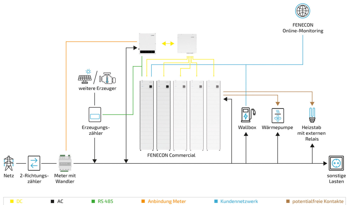
Abbildung 14. Anlage — schematische Darstellung mit optionalen Komponenten (ohne Schutzeinrichtung dargestellt)
