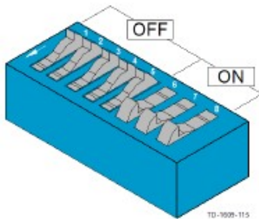
Abbildung 5. DIP-Switch
