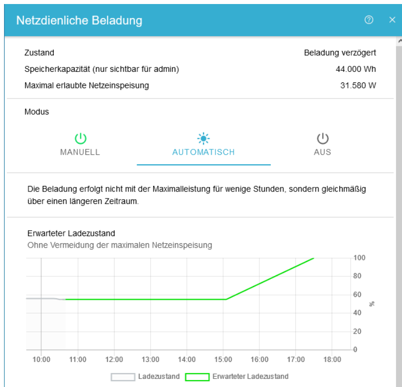
Abbildung 3. Erweiterte Darstellung
