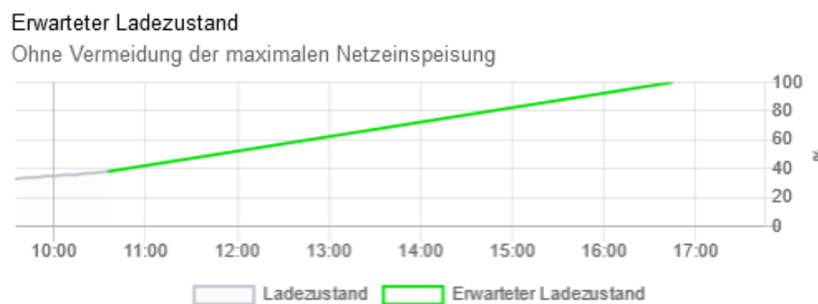
Abbildung 7. Ladezustandsanzeige
