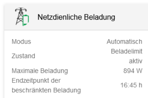
Abbildung 2. Widget Regelbetrieb
