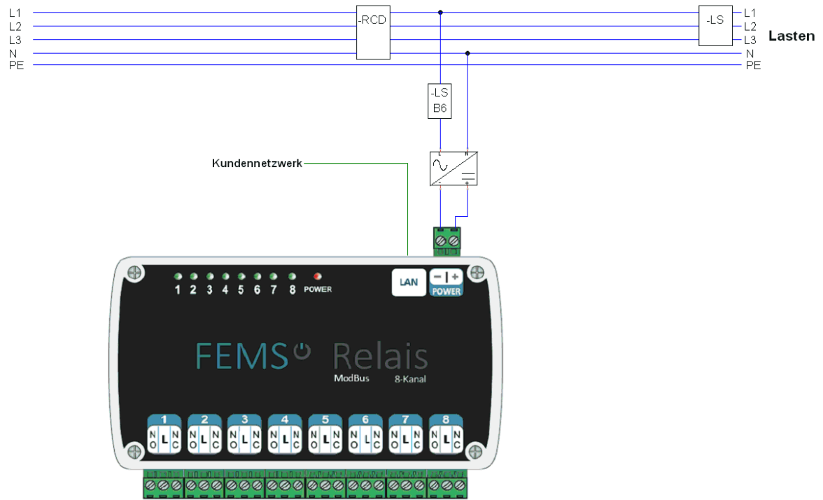
Figure 2. Übersicht FEMS Relaisboard 8-Kanal TCP
