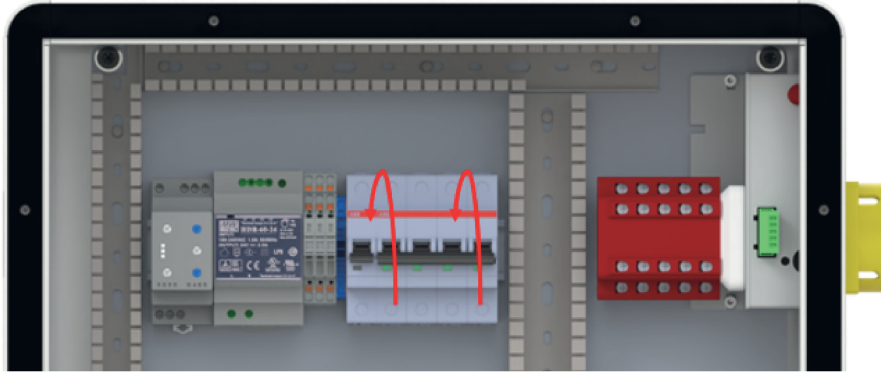
Abbildung 17. Einschalten der Leitungsschutzschalter in der AVU
